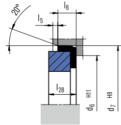
G60 EN 12756
